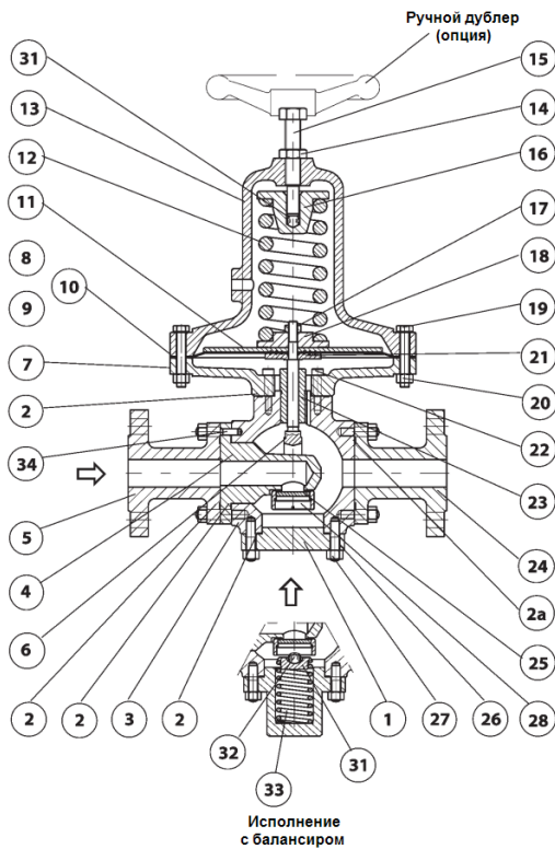
Фланцевое присоединение
