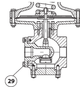
Муфтовое присоединение
